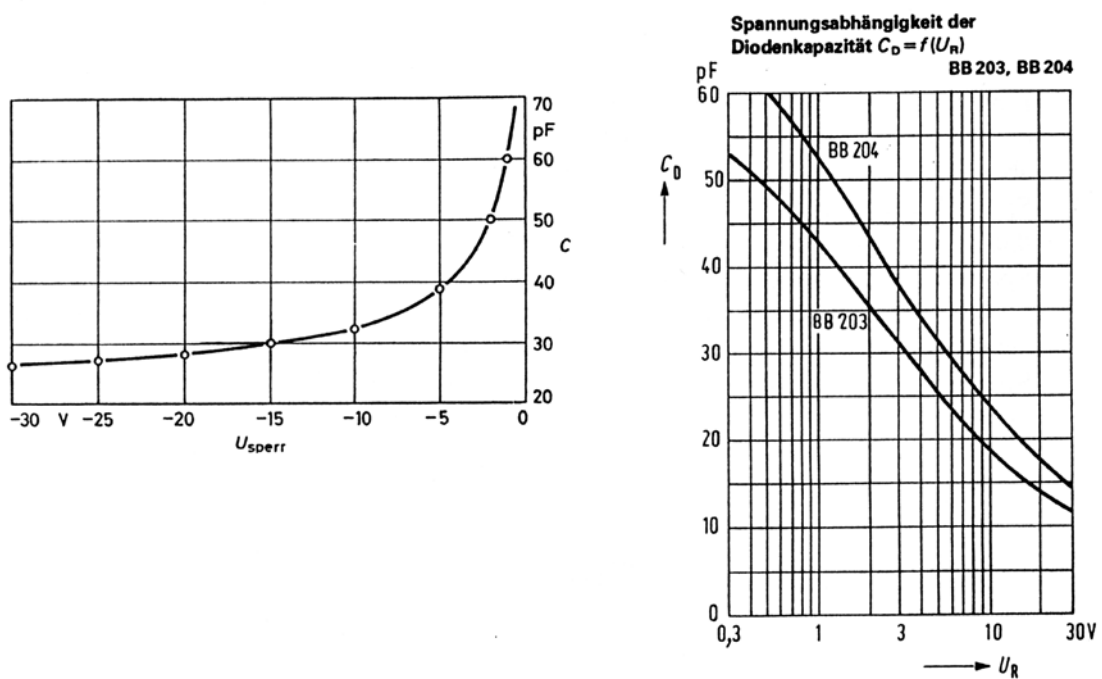
Abb. 1.20 Die Sperrschichtkapazität in Abhängigkeit von der Sperrspannung. Links: linearer, rechts: logarithmischer Maßstab (Quellen: AEG-Telefunken, Siemens).
