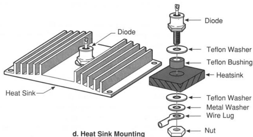
Abb. 1.13 Kühlkörpermontage.
