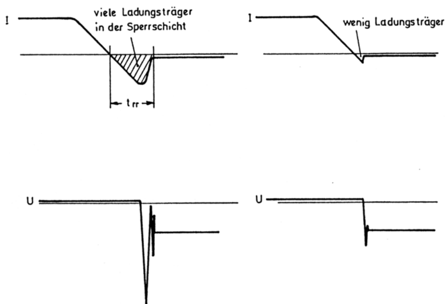
Abb. 1.16 Die Sperrträchtigkeit bei verschiedenen Auslegungen der Sperrschicht.
