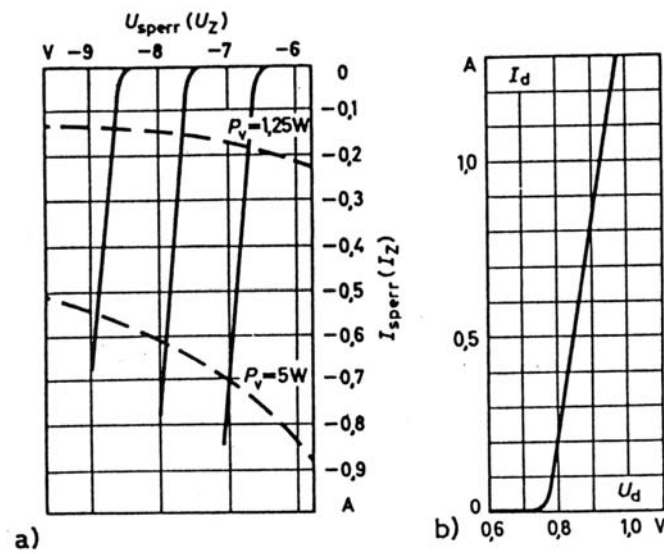
Abb. 1.22 a) Sperr- und b) Durchlaßkennlinien typischer Zenerdioden
