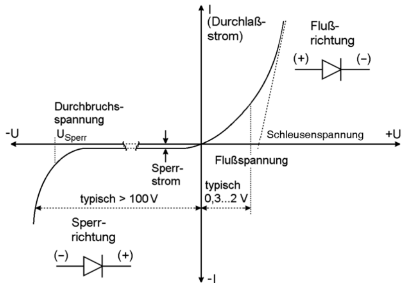
Abb. 1.6 Diodenkennlinie.
