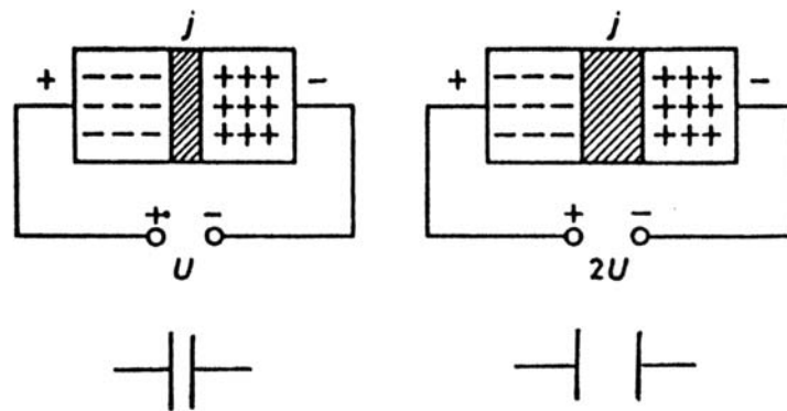
Abb. 1.19 Die Sperrschichtkapazität - das Prinzip der Kapazitätsdiode.
