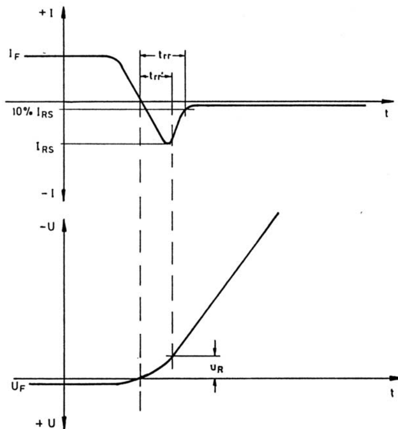
Abb. 1.15 Das Verhalten der Diode beim Umschalten. Oben: der Stromfluß durch die Diode (Durchlaßstrom I_F - Ausräumstrom I_{RS} - Sperrstrom), unten: die Spannung über der Diode (Flußspannung - Sperrspannung).
