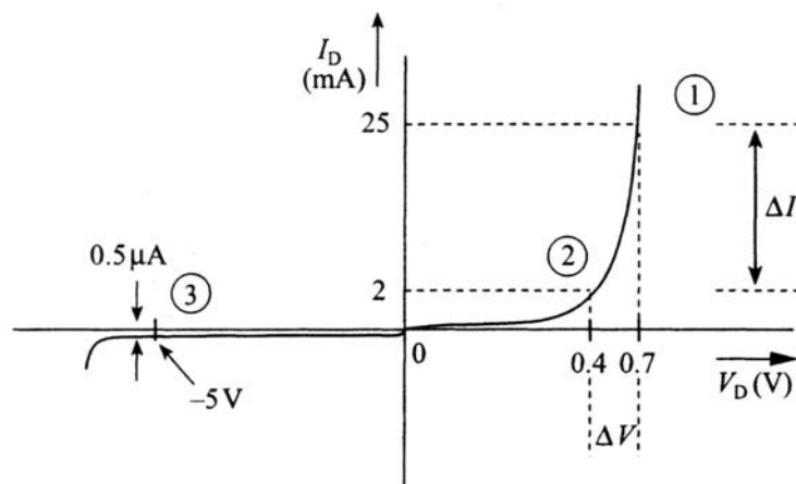
Abb. 1.7 Der statische Widerstand der Diode.
