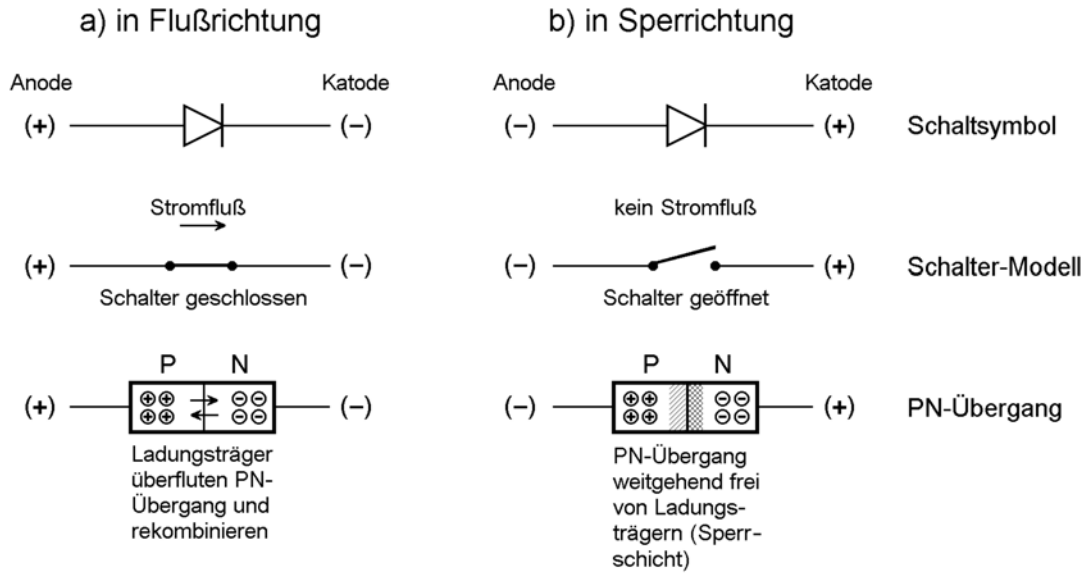
Abb. 1.5 Die (idealisierte) Halbleiterdiode. Die Anode ist P-leitend, die Katode N-leitend.
