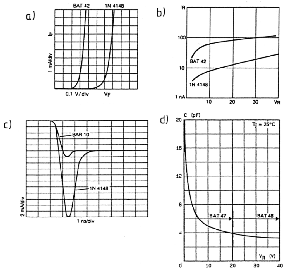
Abb. 1.18 Das statische und dynamische Verhalten von Schottky-Dioden. a) statische Kennlinie in Durchlaßrichtung, b) statische Kennlinie in Sperrichtung, c) Verlauf des Ausräumstromes, d) Sperrschichtkapazität in Abhängigkeit von der Sperrspannung (Quelle: SGS-Thomson).
