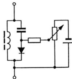
Abb. 1.21 Schwingkreis-Abstimmung mittels Kapazitätsdiode.
